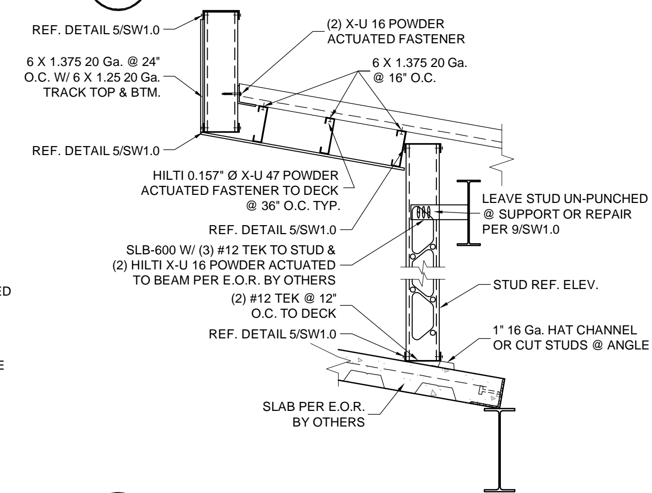
15 WALL ON ROOF N.T.S.
