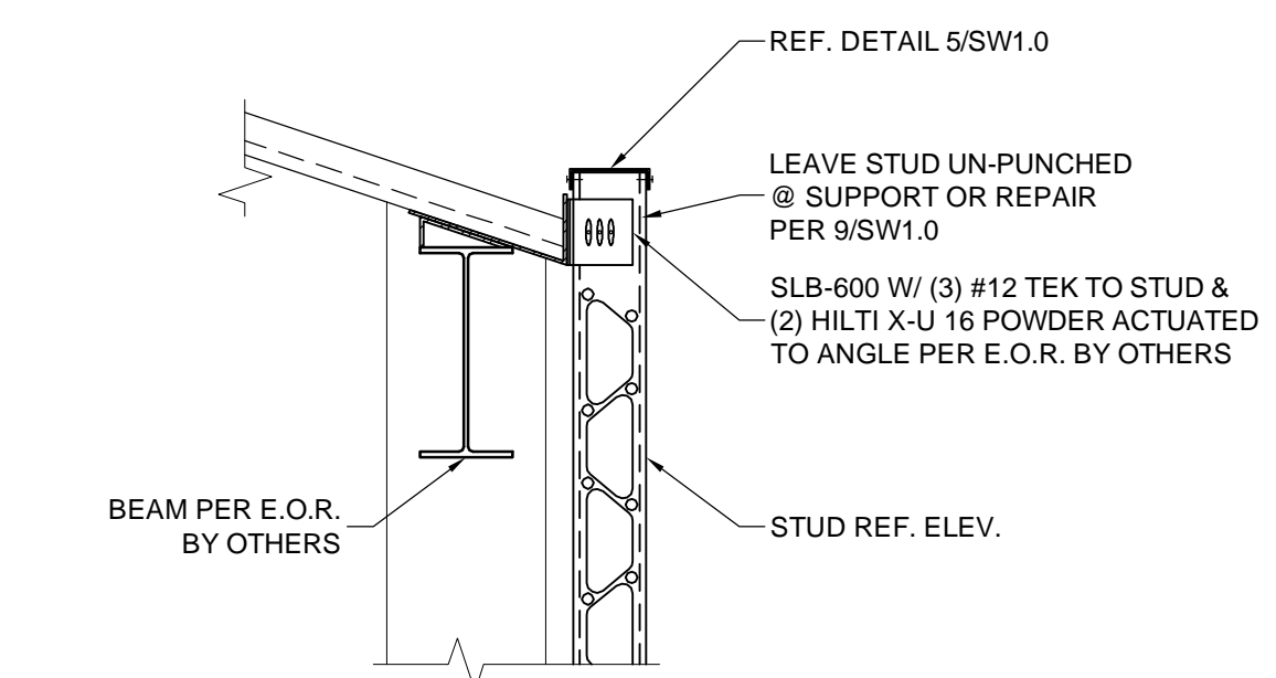
15 WALL ON ROOF N.T.S.
