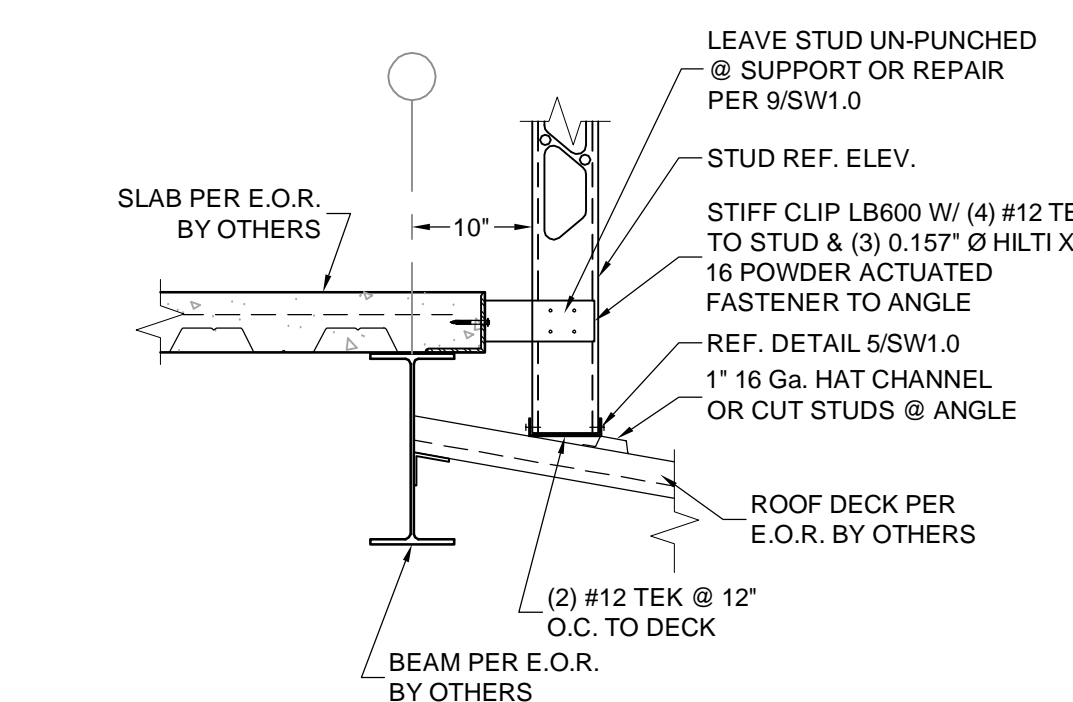
18 STUD TO DECK N.T.S.
